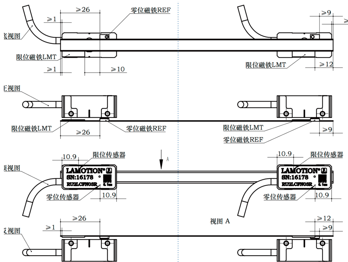
栅尺左端安装零位磁铁
