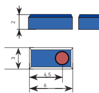
原点磁铁 RU2-REF-M
