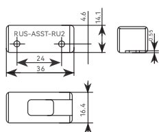
贴尺工具 RUS-ASST-RU2
